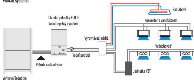
Venkovní jednotka
