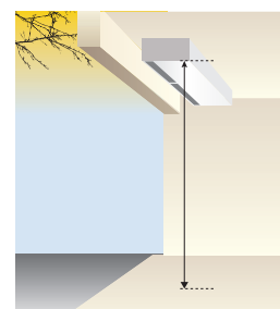
Maximální výška instalace. Tryskové proudění: 3,5 m Standardní proudění: 3,0 m
